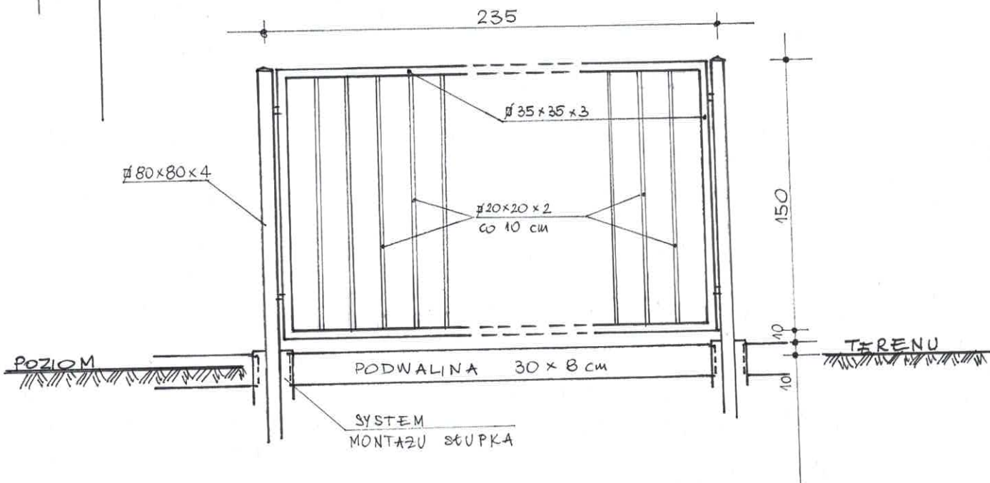
SCHEMAT PRZEŚCIA
